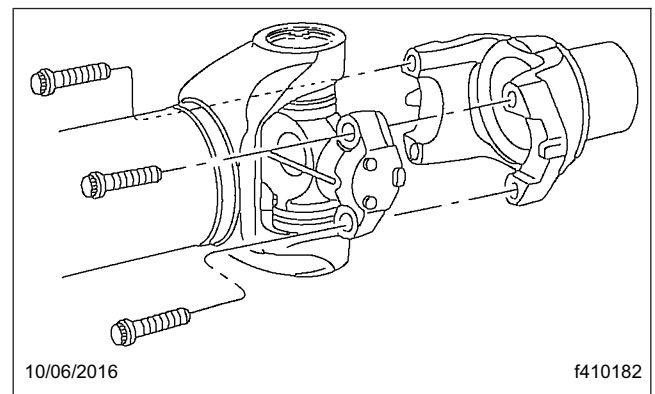
Figura 2, Juntas universales Meritor serie RPL, excepto RPL35
