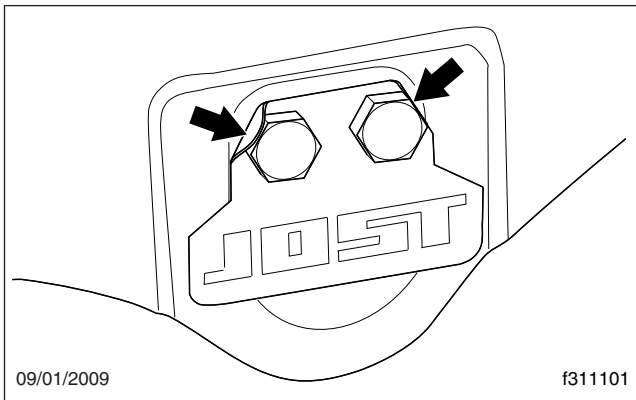
Figura 3, Lengüetas de seguridad de los pernos de los pasadores de los soportes
