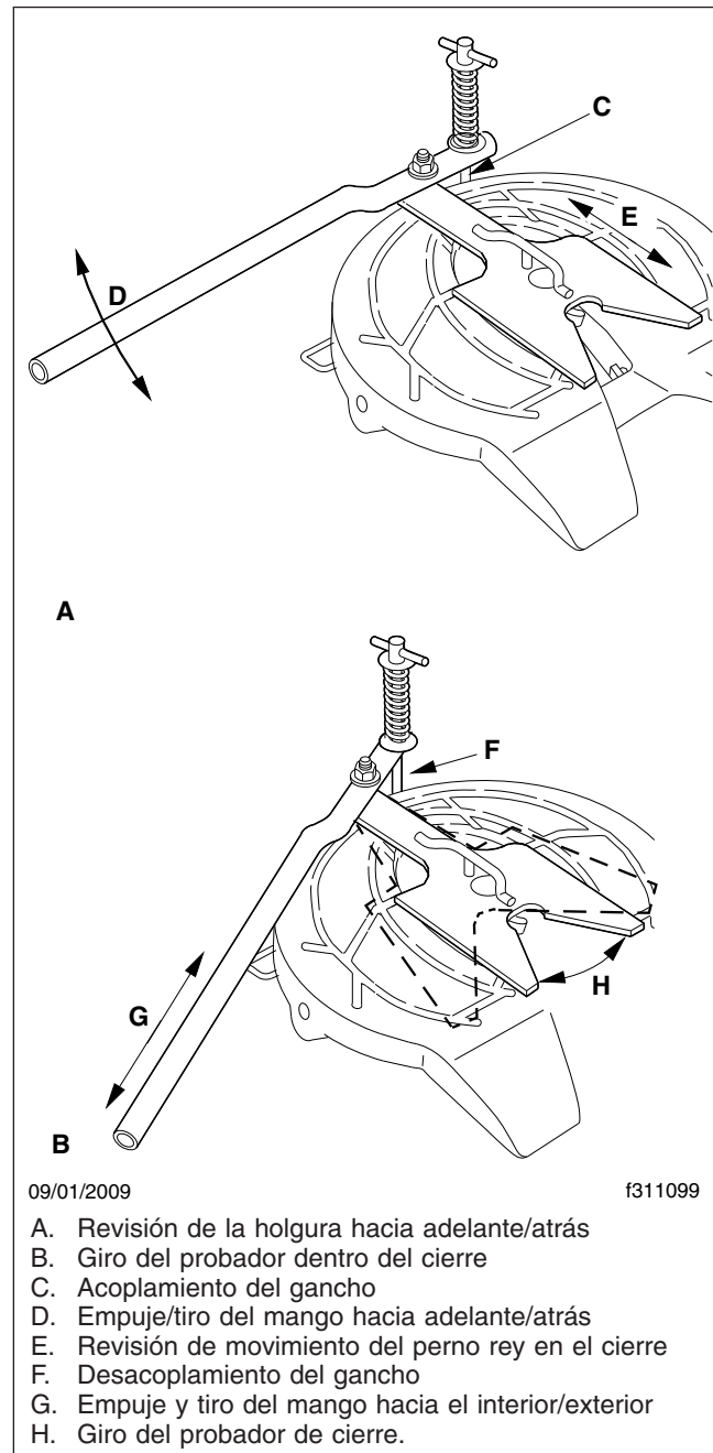
Figura 4, Ajuste de la quinta rueda Jost
