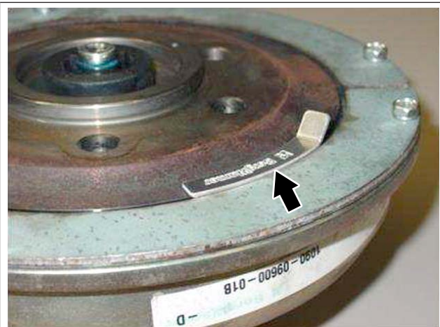
Figura 4, Placa de retención abajo de la herramienta, aún hay vida útil
