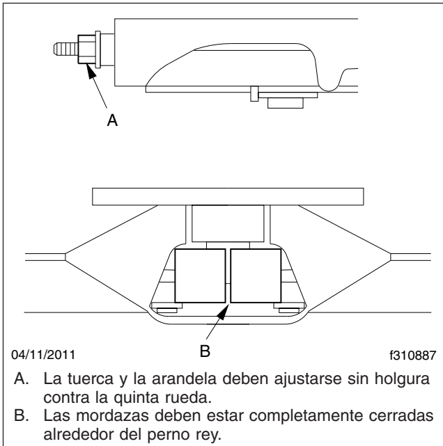
Figura 1, Quinta rueda Holland cerrada correctamente
