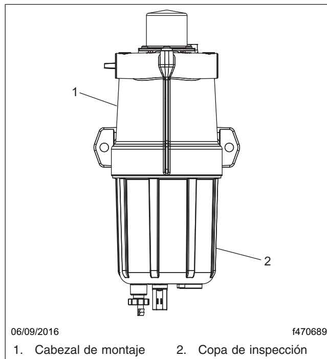
Figura 1, Separador de combustible y agua Detroit
