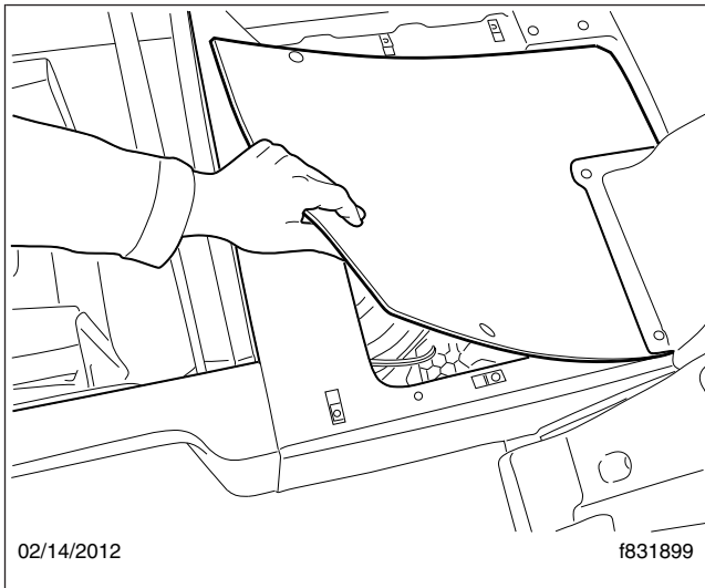
Figura 6, Panel de acceso al sistema HVAC del dormitorio de 48 pulgadas
