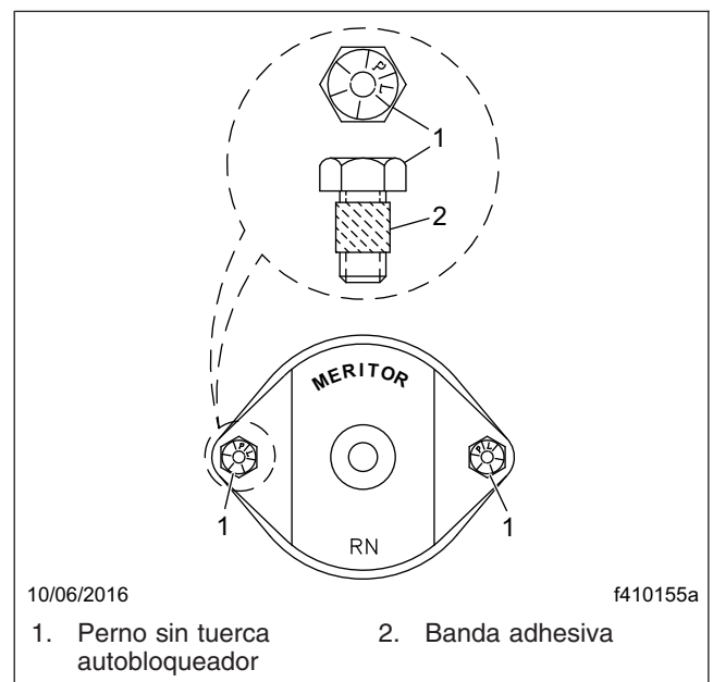
Figura 1, Sujetadores de juntas universales Meritor para las tapas de cruceta
