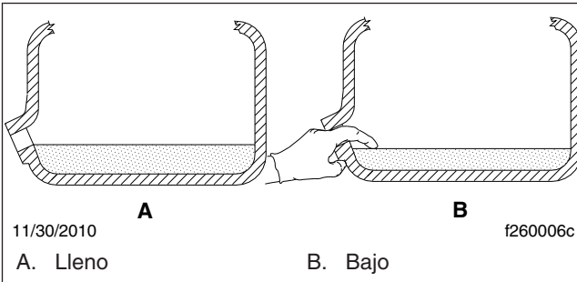
Figura 3, Revisión del nivel de líquido para transmisión
