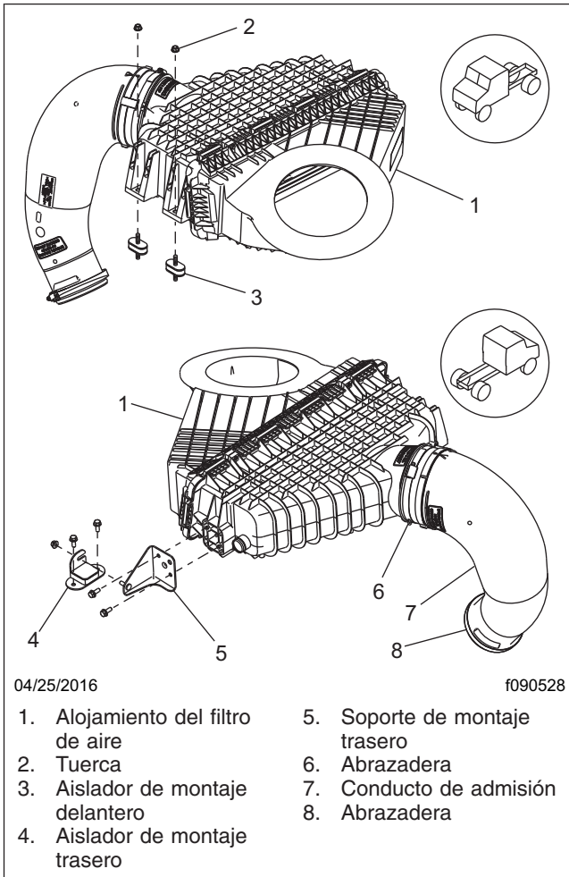
Figura 3, Ensamble del filtro de aire
