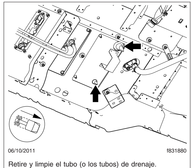
Figura 10, Inspección del tubo de drenaje
