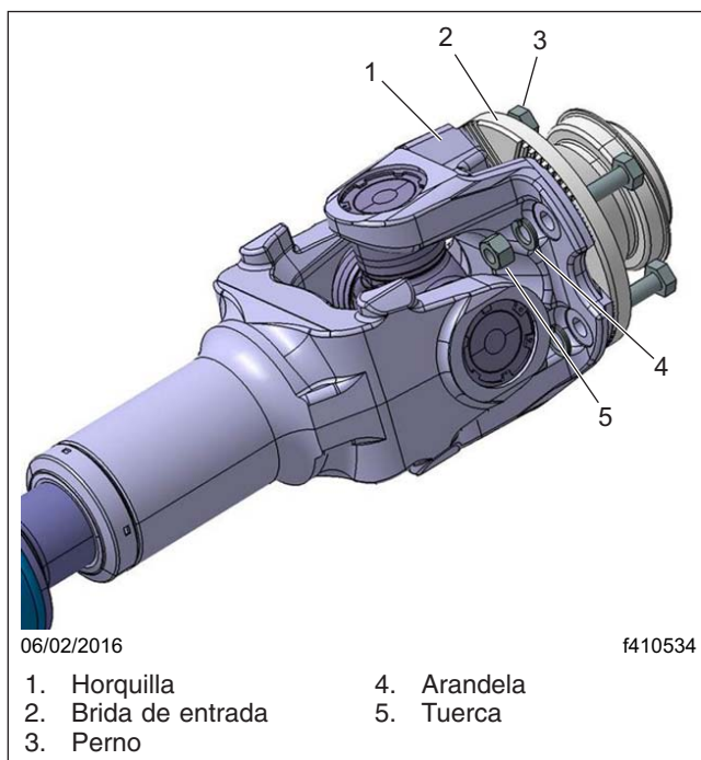
Figura 4, Junta universal Meritor serie RPL35
