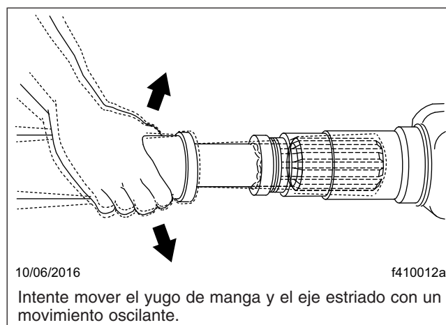
Figura 5, Revisión del desgaste de las estrías de la junta deslizable
