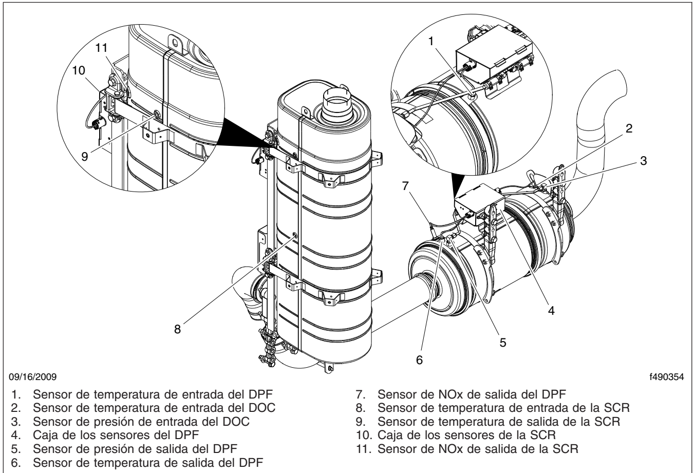
Figura 3, Ubicaciones de los sensores del ATS de dos unidades 2HV
