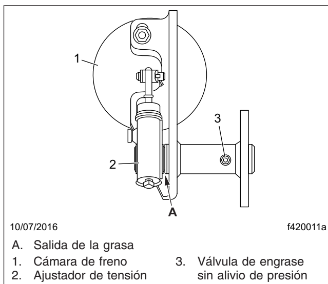
Figura 6, Lubricación del soporte del eje de levas
