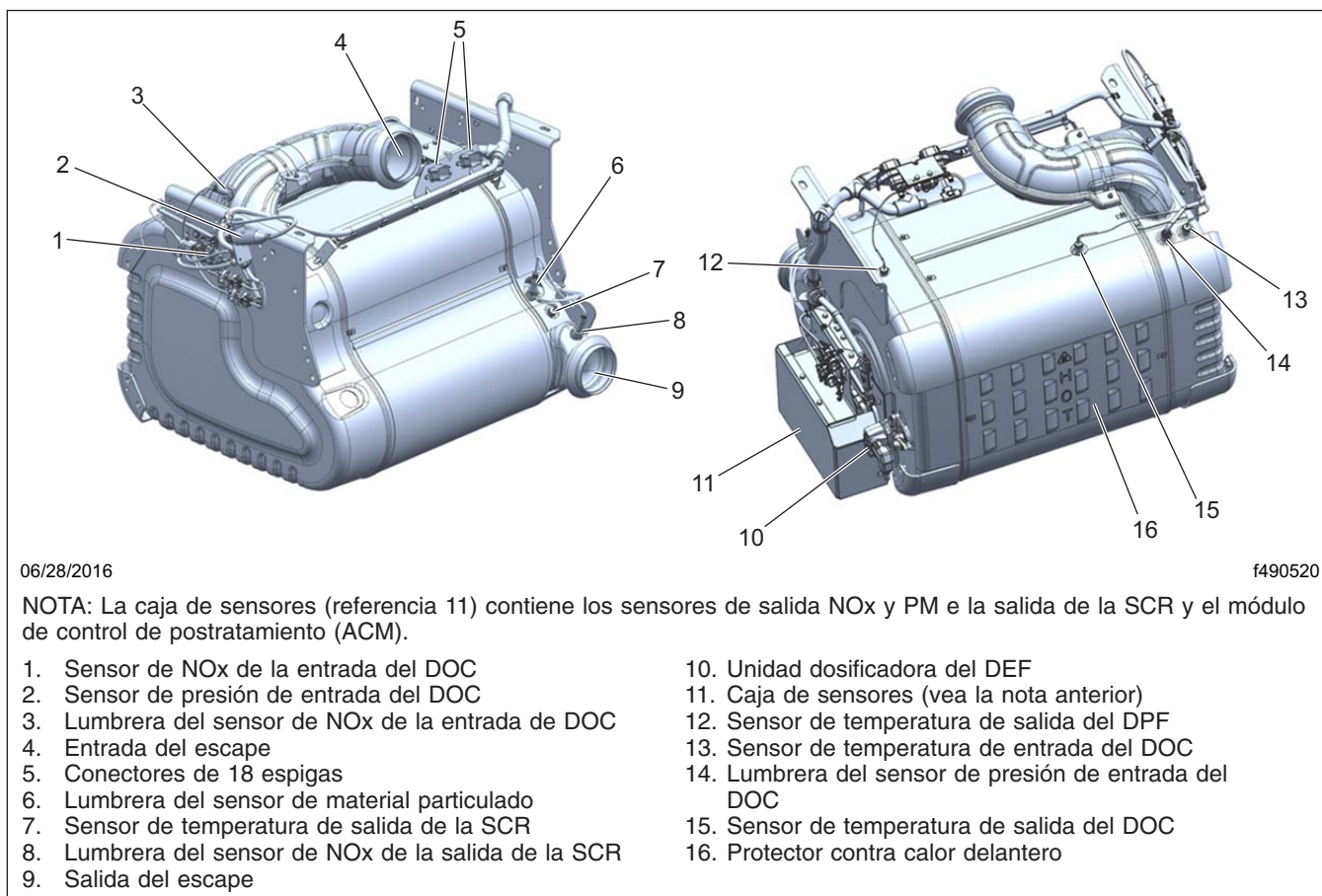
Figura 1, Ubicaciones de los sensores del ATS de una sola unidad
