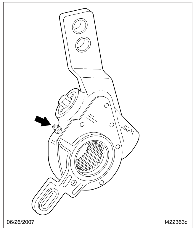
Figura 5, Válvula de engrase del ajustador de tensión automático Haldex
