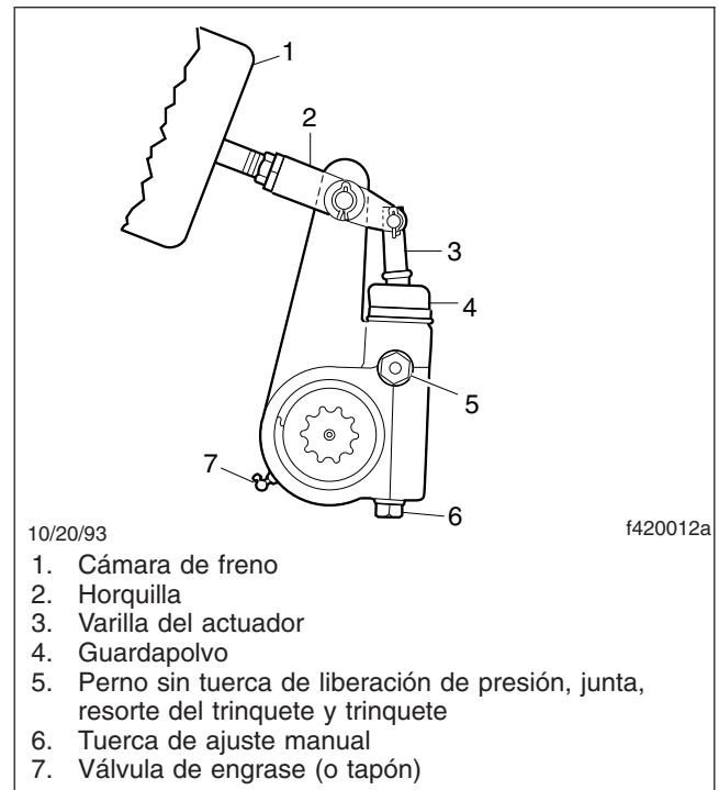
Figura 7, Ajustador de tensión automático Meritor
