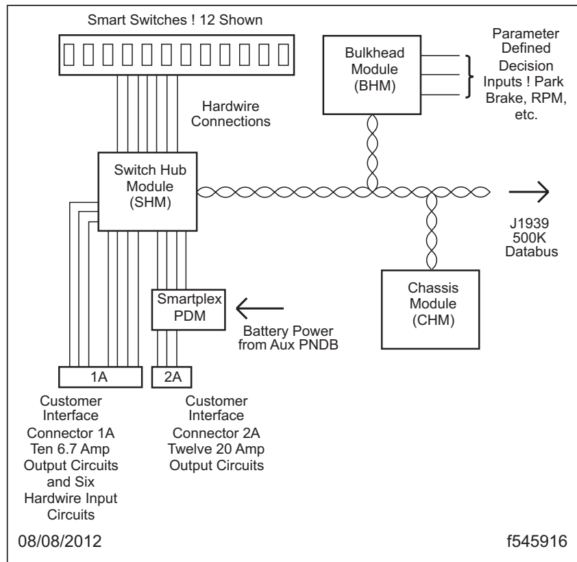
SmartplexSystemDiagram
