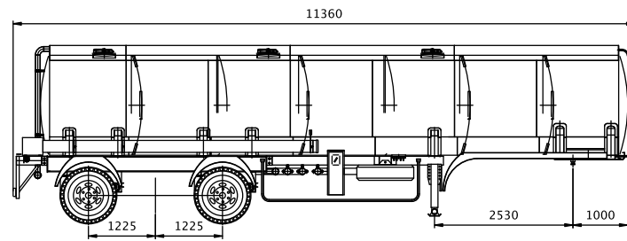
Semiremolque para Transporte de Combustible 35 m3
