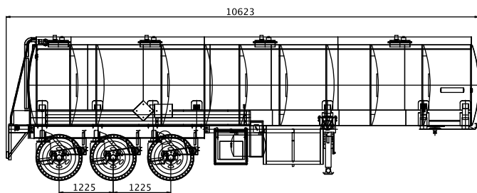
Semiremolque para Transporte de Combustible 33 m3
